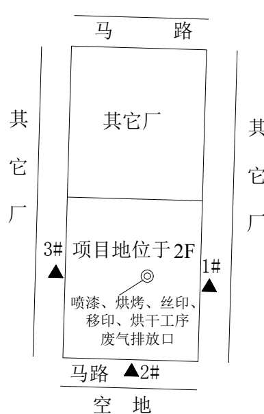
图 3-2 厂区平面布置及监测点位
