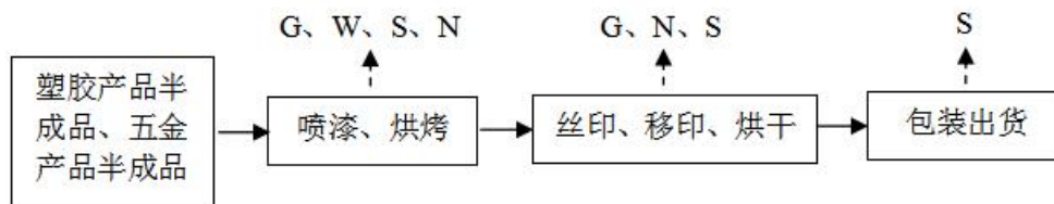
图 3-3 项目塑胶产品、五金产品生产工艺及产污环节流程图
