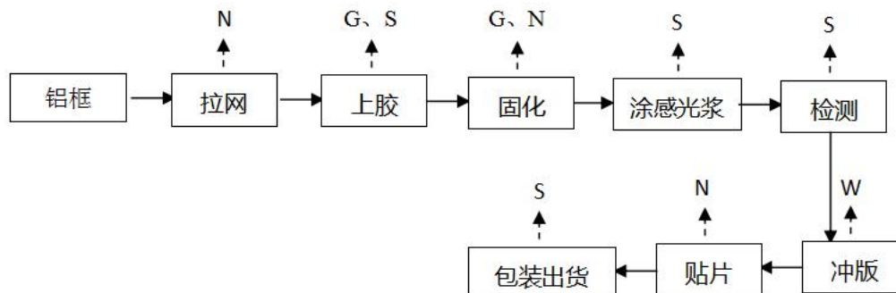
图 3-3 网版生产工艺及产污环节图
